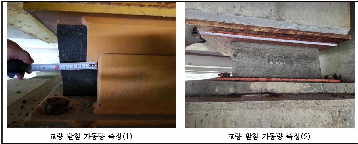
【사진 18.3.43】 교량받침 이동량 측정
