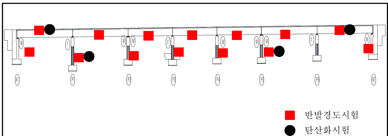
【그림 18.4.1】 상주방향 콘크리트 내구성조사 위치도
