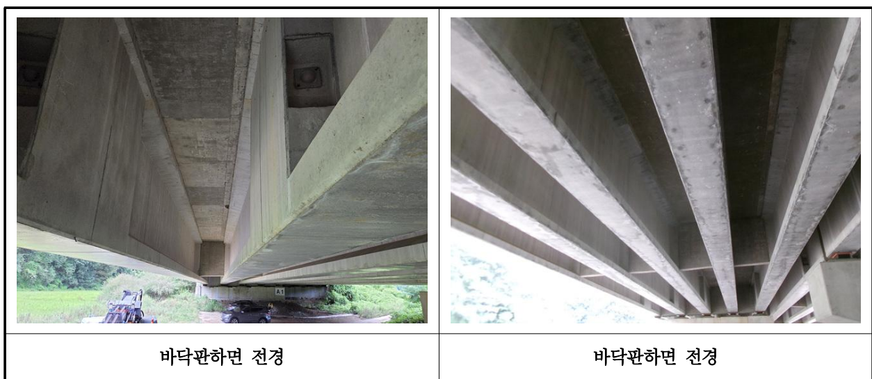
【사진 18.3.29】 바닥판하면 전경
