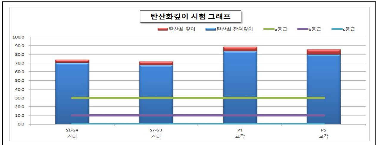
【그림 18.4.7】 상주방향 탄산화 깊이 측정결과
