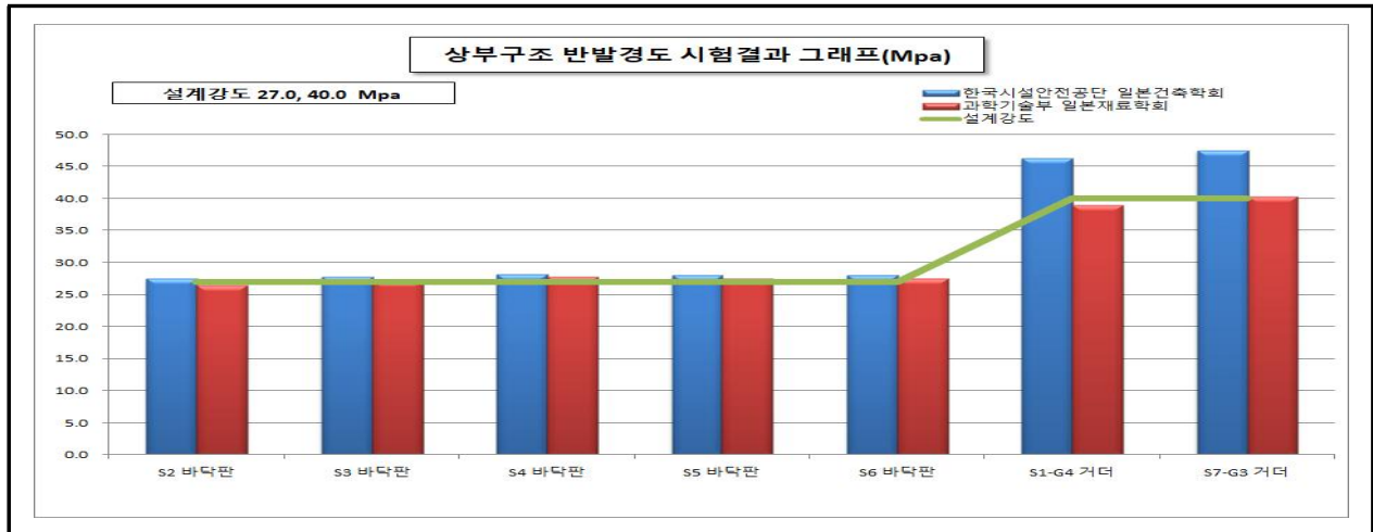
【그림 18.4.3】 상주방향 상부구조 반발경도시험 측정결과
