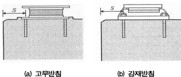
【그림 18.3.2】 도로교설계기준 연단거리 산출방법
