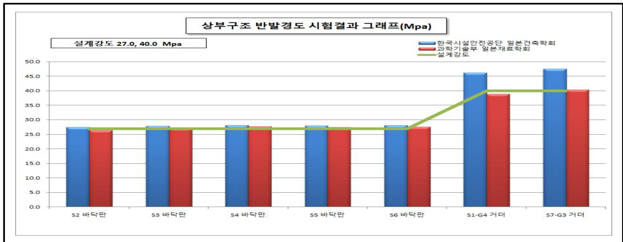
【그림 18.4.5】 영천방향 상부구조 반발경도시험 측정결과
