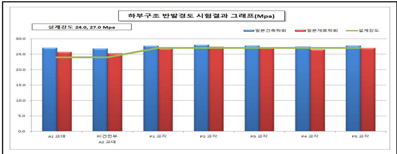
【그림 18.4.4】 상주방향 하부구조 반발경도시험 측정결과
