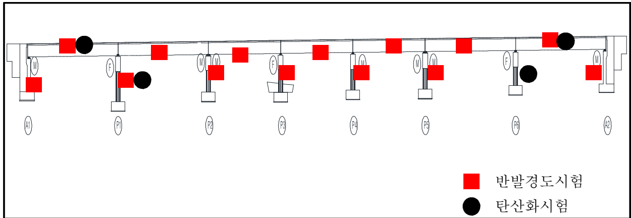
【그림 18.4.2】 영천방향 콘크리트 내구성조사 위치도
