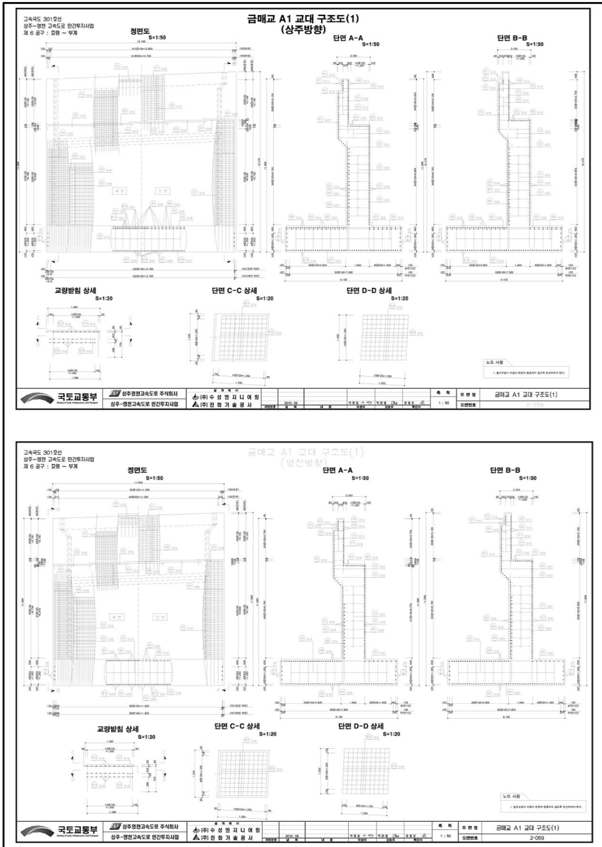
【그림 18.1.9】 교대 배근도
