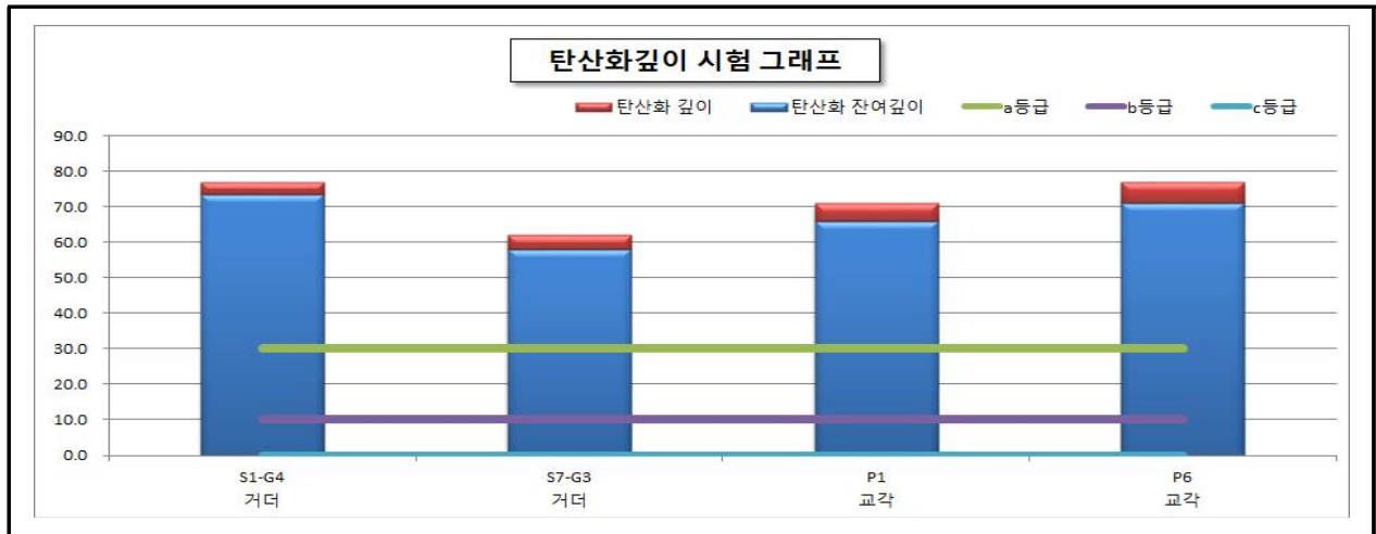
【그림 18.4.8】 영천방향 탄산화 깊이 측정결과
